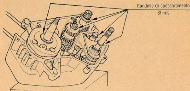
FIG. 25 Interno motore Engine inside
