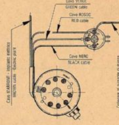
FIG. 7 Schema collegamento fili Wiring diagram
