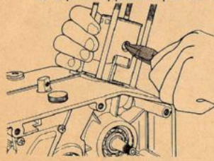
FIG. 20 Rimozione anelli di fermo Securing ring removal
