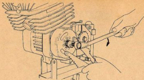
FIG. 10 Estrazione girante volano Flywheel magnet rotor pulling
