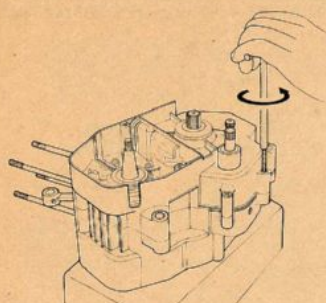
FIG. 22 Rimozione viti Screw removal
