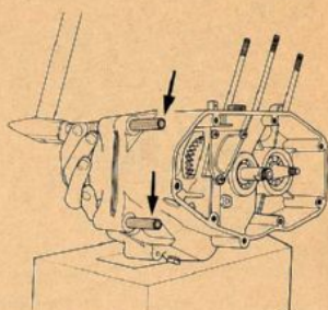
FIG. 23 Rimozione grani Dowels removal
