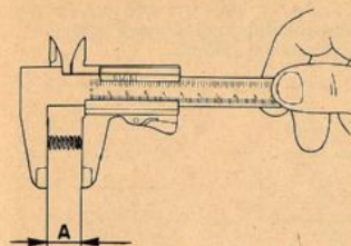
FIG. 33 Controllo molle frizione Clutch spring check
