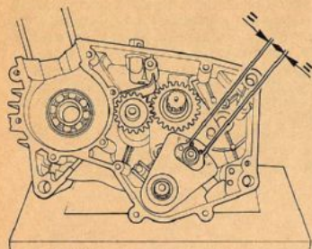
FIG. 40 Posizione di montaggio selettore Selector assembly position
