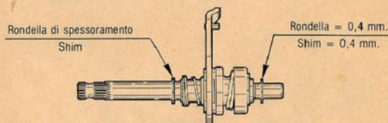
FIG. 32 Gruppo selettore Gear-box selector
