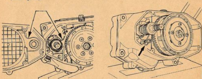
FIG. 50 Montaggio gruppo avviamento Start assembly
