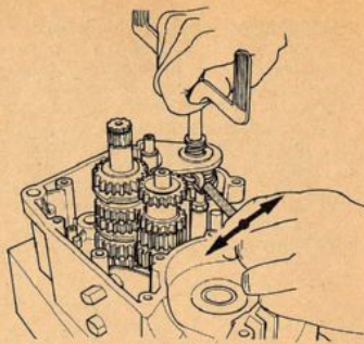
FIG. 41 Registrazione selettore Selector adjustment
