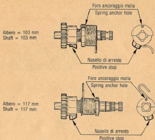
FIG. 49 Controllo fase gruppo avviamento Start stroke check
