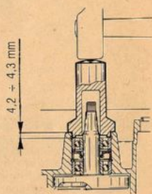
FIG. 46 Montaggio cuscinetto Bearing assembly
