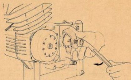
FIG. 14 Estrazione pignone catena Chain sprocket pulling
