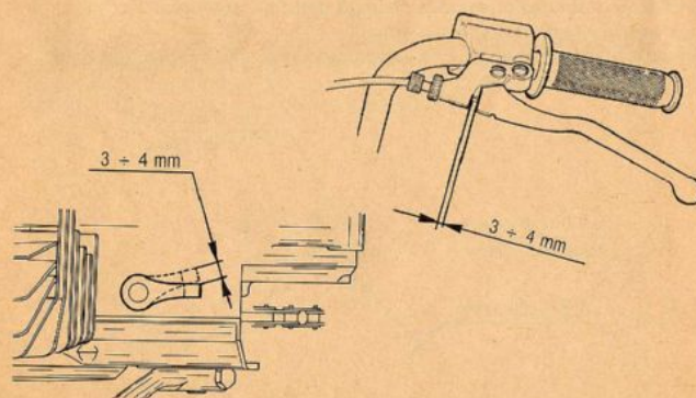
FIG. 4 Controllo gioco frizione Clutch clearance check
