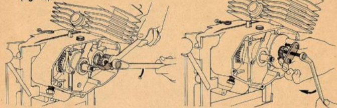
FIG. 19 Estrazione pignone motore Pinion pulling
