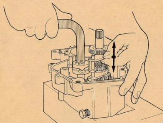
FIG. 39 Controllo cambio Gear-box check
