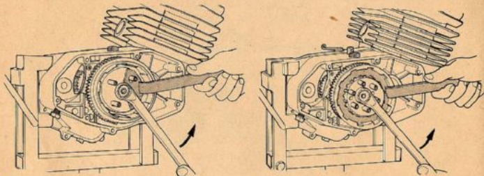
FIG. 17 Rimozione dado Nut removal
