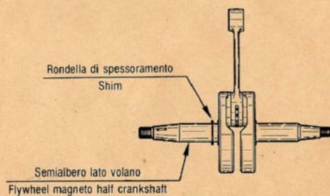
FIG. 29 Imbiellaggio Crankshaft
