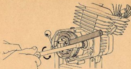
FIG. 16 Rimozione dado pignone motore Pinon nut removal
