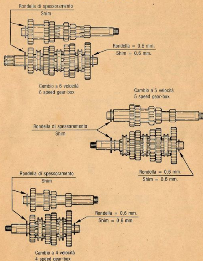
FIG. 30 Cambio Gear-box
