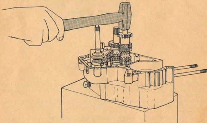
FIG. 42 Montaggio albero primario Primary shaft assembly
