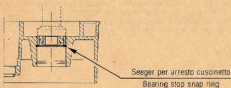
FIG. 28 Montaggio cuscinetto banco «P6» «P6» crankshaft bearing assembly
