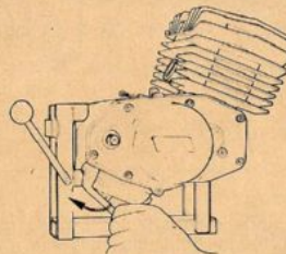
FIG. 15 Rimozione vite Screw removal
