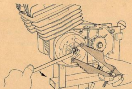
FIG. 9 Rimozione dado volano Flywheel magneto nut removal
